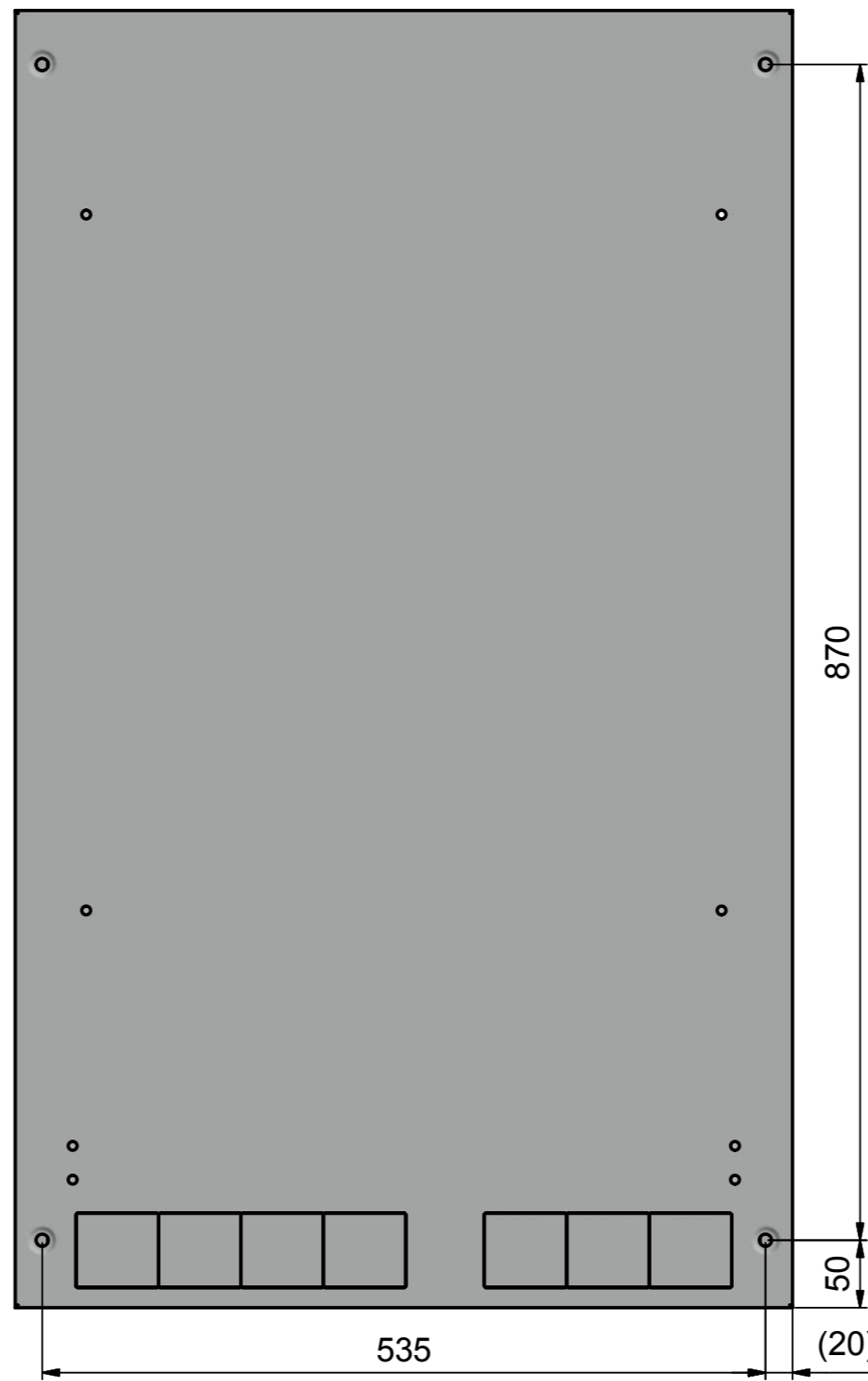
Befestigungspunkte Wand
