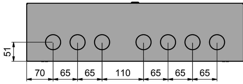
Rohraussparungen unten
