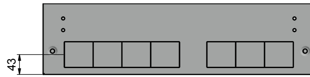
Rohraussparungen hinten
